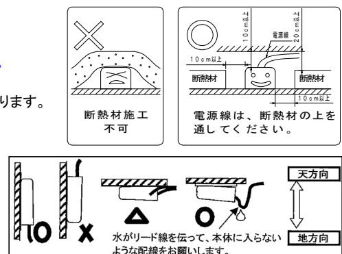
LED専用電源の設置図
