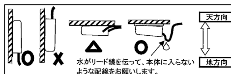
LED専用電源の設置図
