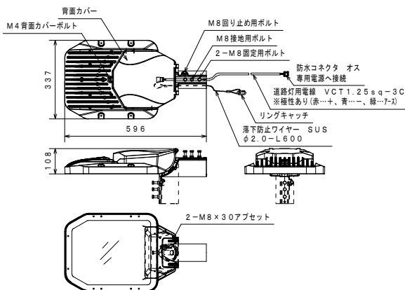
図 照明器具背面カバー内 詳細
