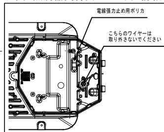
図 照明器具背面カバー内 詳細
