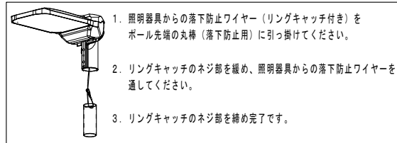
図 落下防止ワイヤー取付手順(チョーク吊り)
