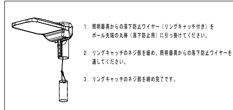
図 落下防止ワイヤー取付手順(チョーク吊り)
