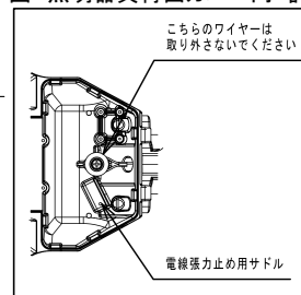
図 照明器具背面カバー内 詳細
